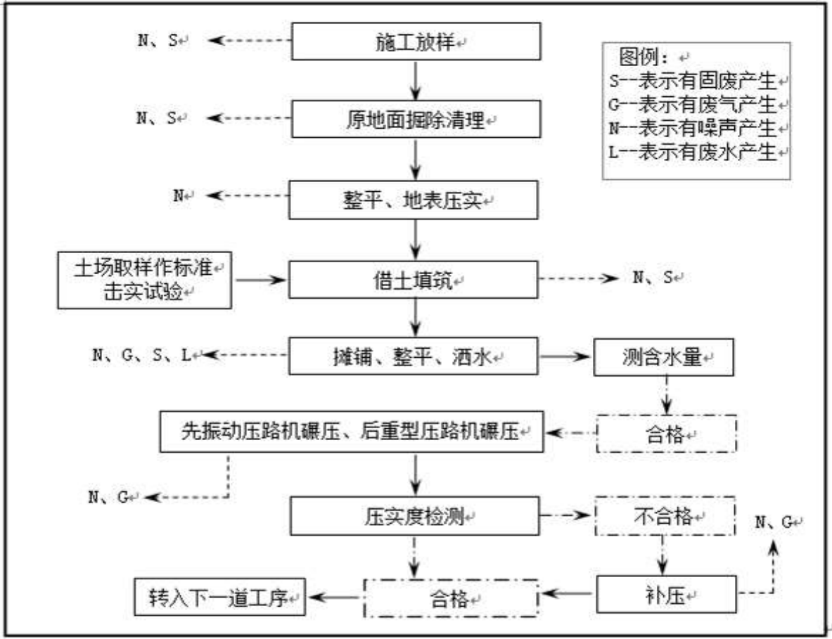
图 2.10-1 路基填筑施工工艺及产污环节框图
