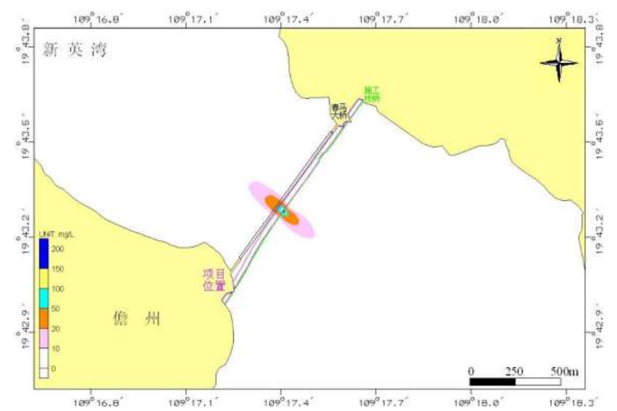
图 4.6-2 源强点 A 桩基施工过程中悬浮泥沙增量分布最大包络线图
