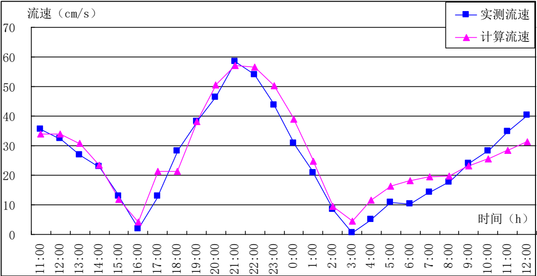
图 4.3-4 3#站潮流流速流向验证曲线(2020 年 9 月 15 日 ~ 16 日)
