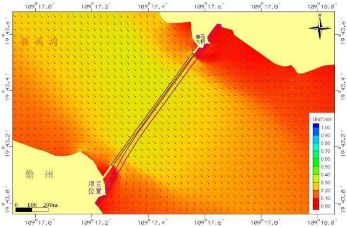
图 4.3-9 工程前项目工程用海区域涨急流场
