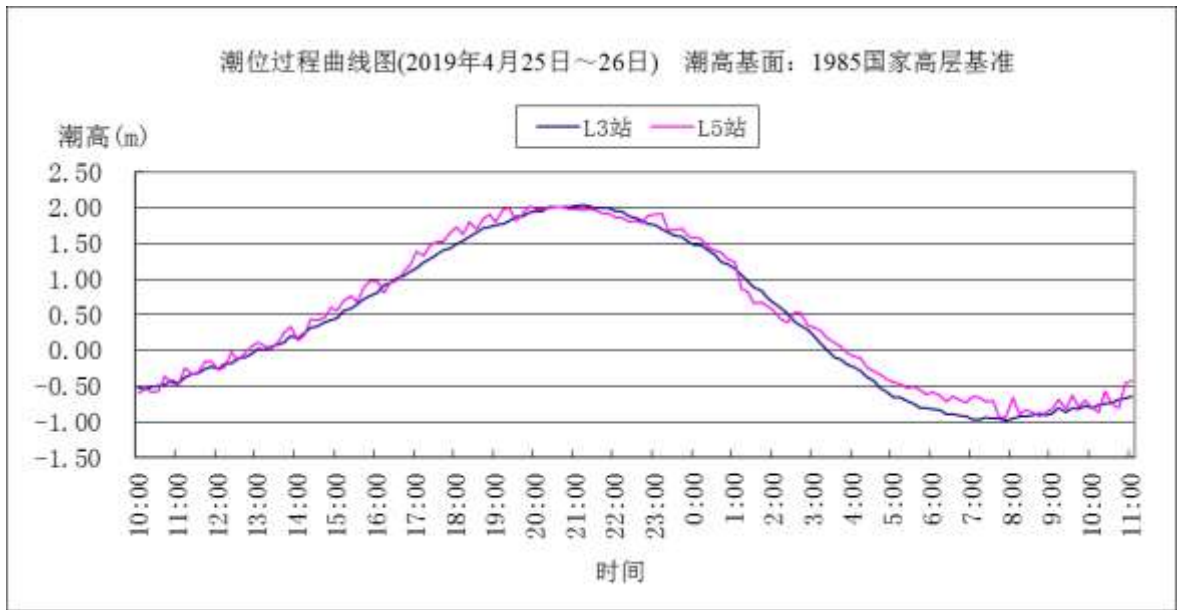
图 3.4-1 2019 年春季观测期间潮位过程曲线图
