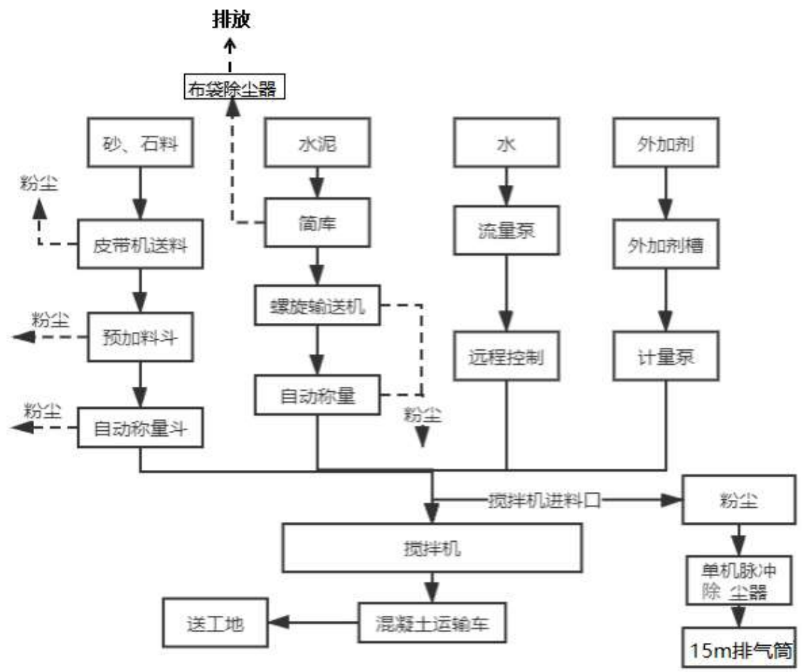
水泥混凝土搅拌站生产工艺流程及产污环节图
