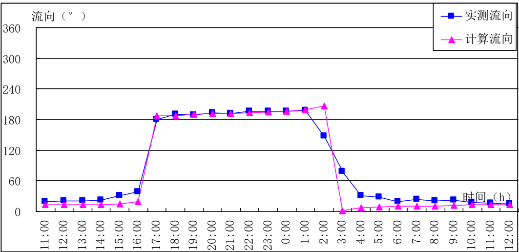
图 4.3-6 5#站潮流流速流向验证曲线(2020 年 9 月 15 日 ~ 16 日)
