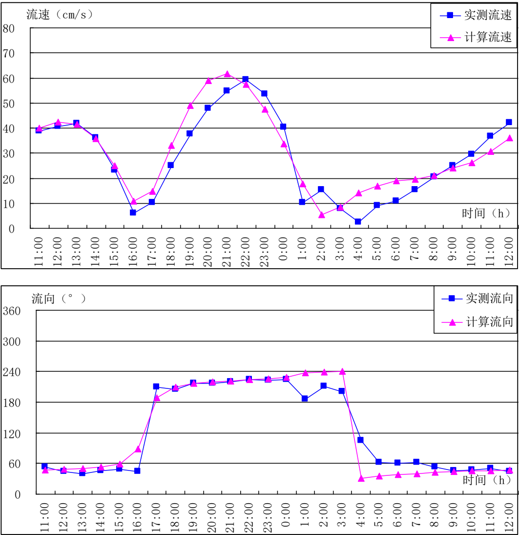
图 4.3-7 6#站潮流流速流向验证曲线(2020 年 9 月 15 日 ~ 16 日)
