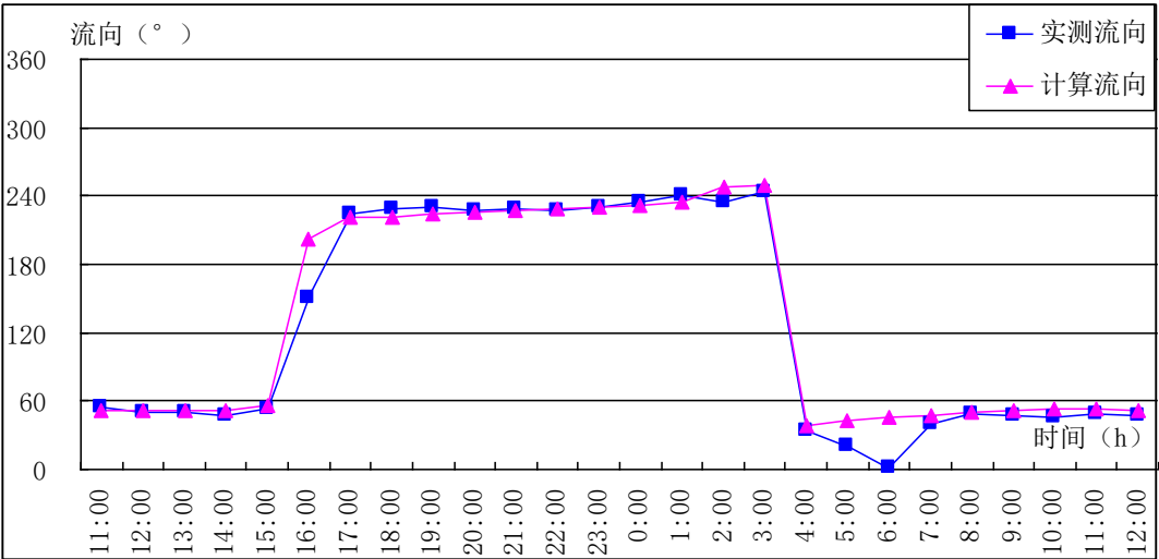
图 4.3-5 4#站潮流流速流向验证曲线(2020 年 9 月 15 日 ~ 16 日)
