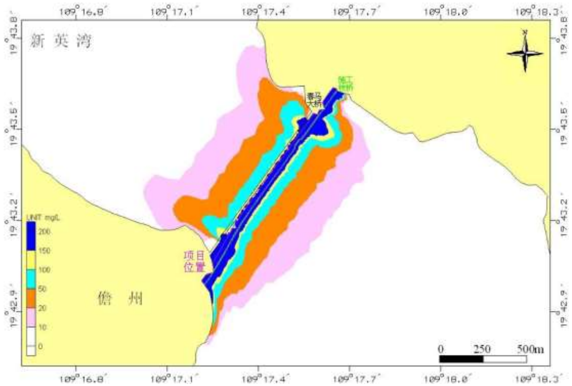
图 4.6-10 四种工况叠加后的悬浮泥沙增量分布最大包络线图
