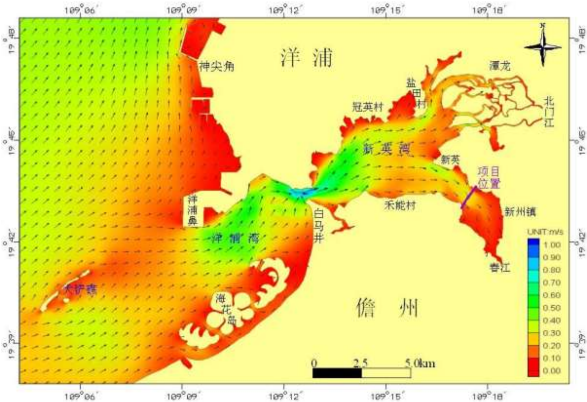
图 4.3-8 工程前项目工程附近海域涨急流场
