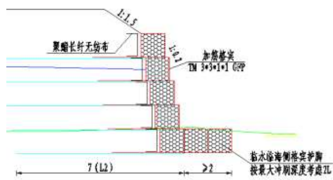
临海、水田、低洼地段落路肩墙防护
