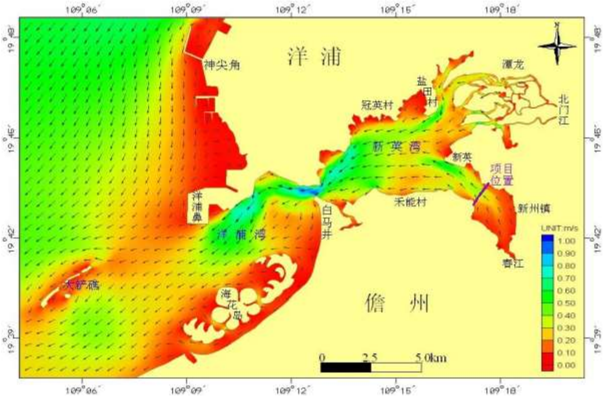
图 4.3-10 工程前项目工程附近海域落急流场
