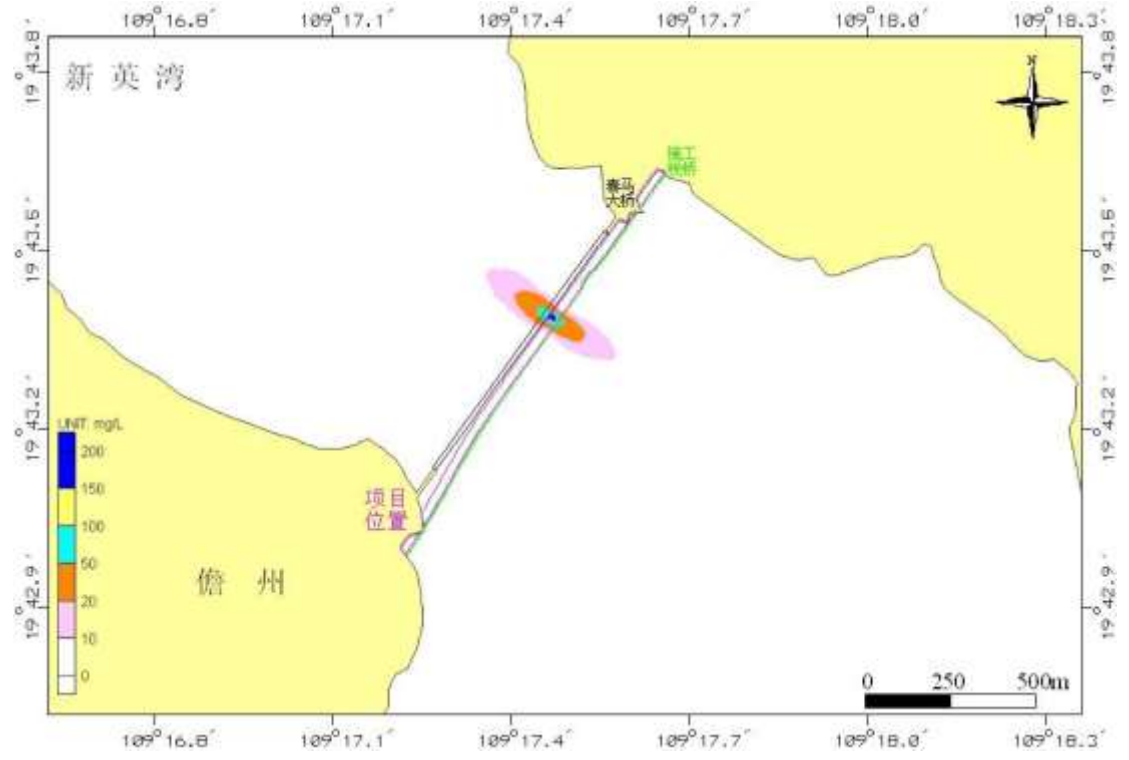
图 4.6-4 源强点 B 围堰施工过程中悬浮泥沙增量分布最大包络线图
