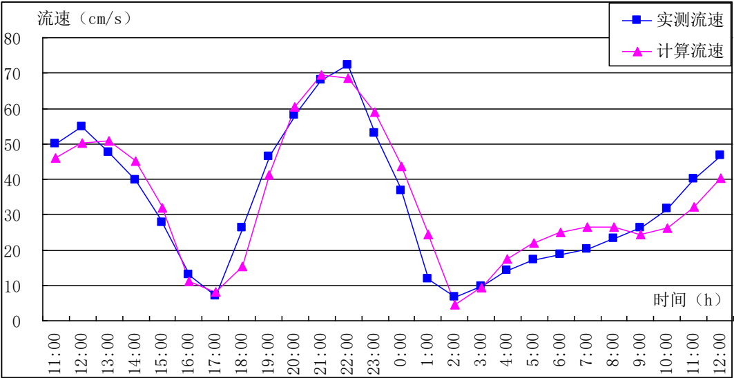
图 4.3-5 4#站潮流流速流向验证曲线(2020 年 9 月 15 日 ~ 16 日)
