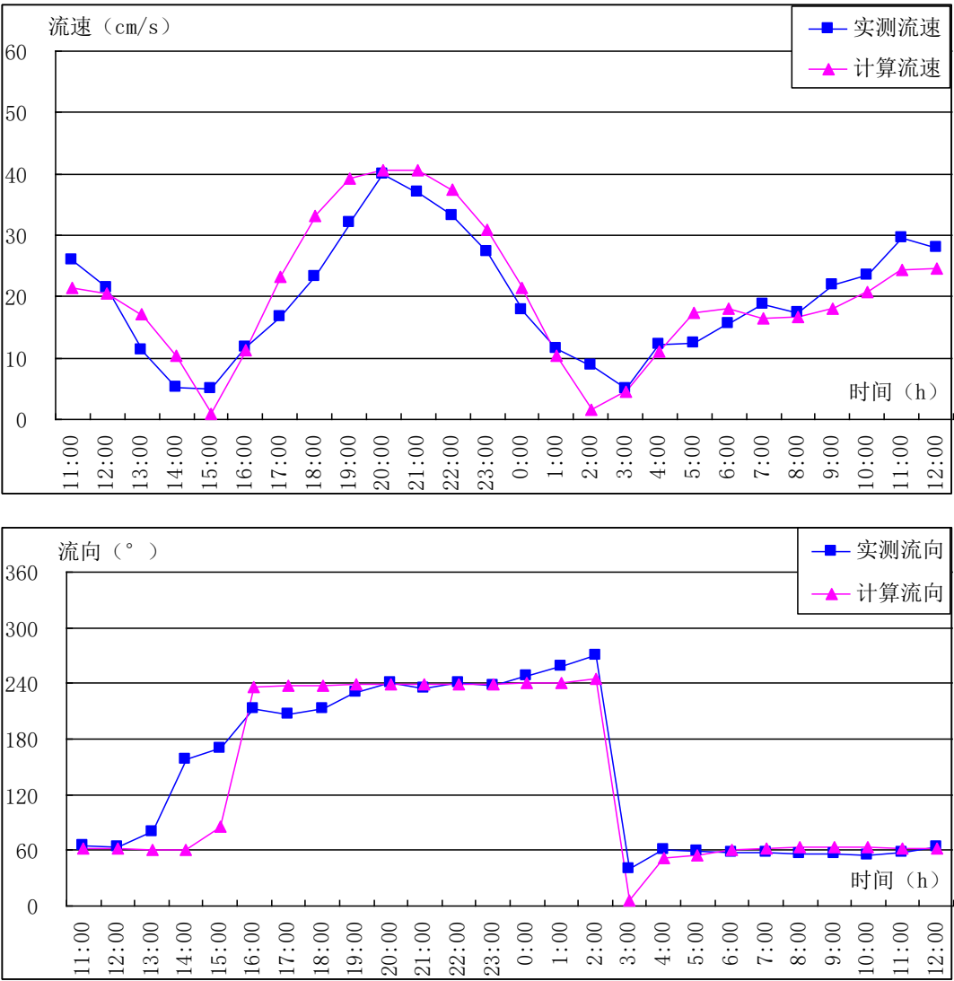
图 4.3-4 3#站潮流流速流向验证曲线(2020 年 9 月 15 日 ~ 16 日)
