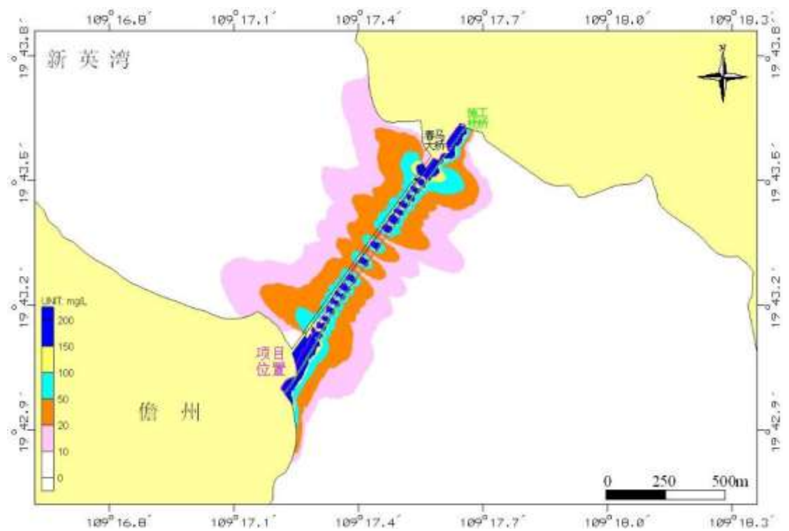
图 4.6-5 整个钢板桩围堰施工过程中悬浮泥沙增量分布最大包络线图
