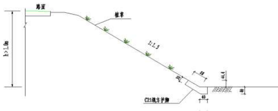
填方边坡植草防护
