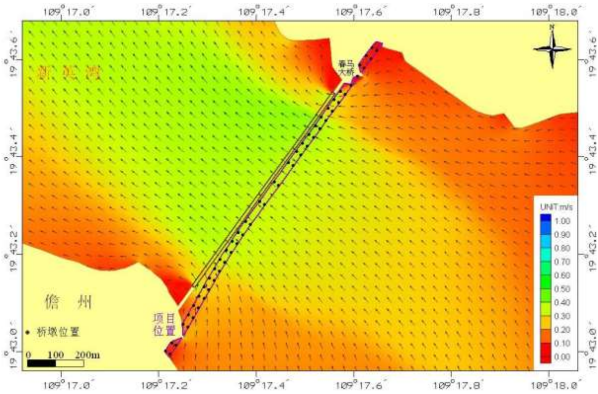
图 4.3-13 工程后项目工程用海区域落急流场
