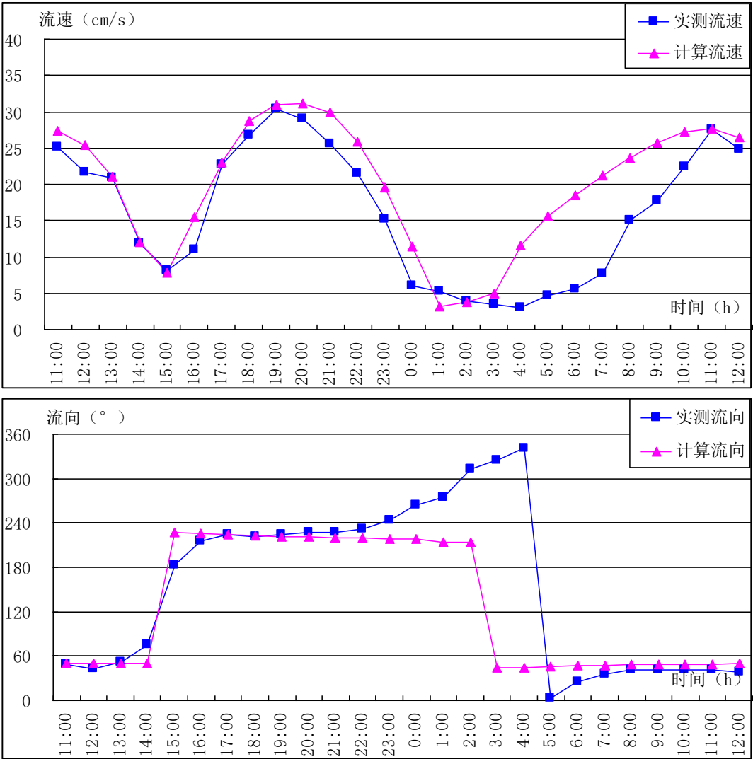
图 4.3-3 2#站潮流流速流向验证曲线(2020 年 9 月 15 日~16 日)
