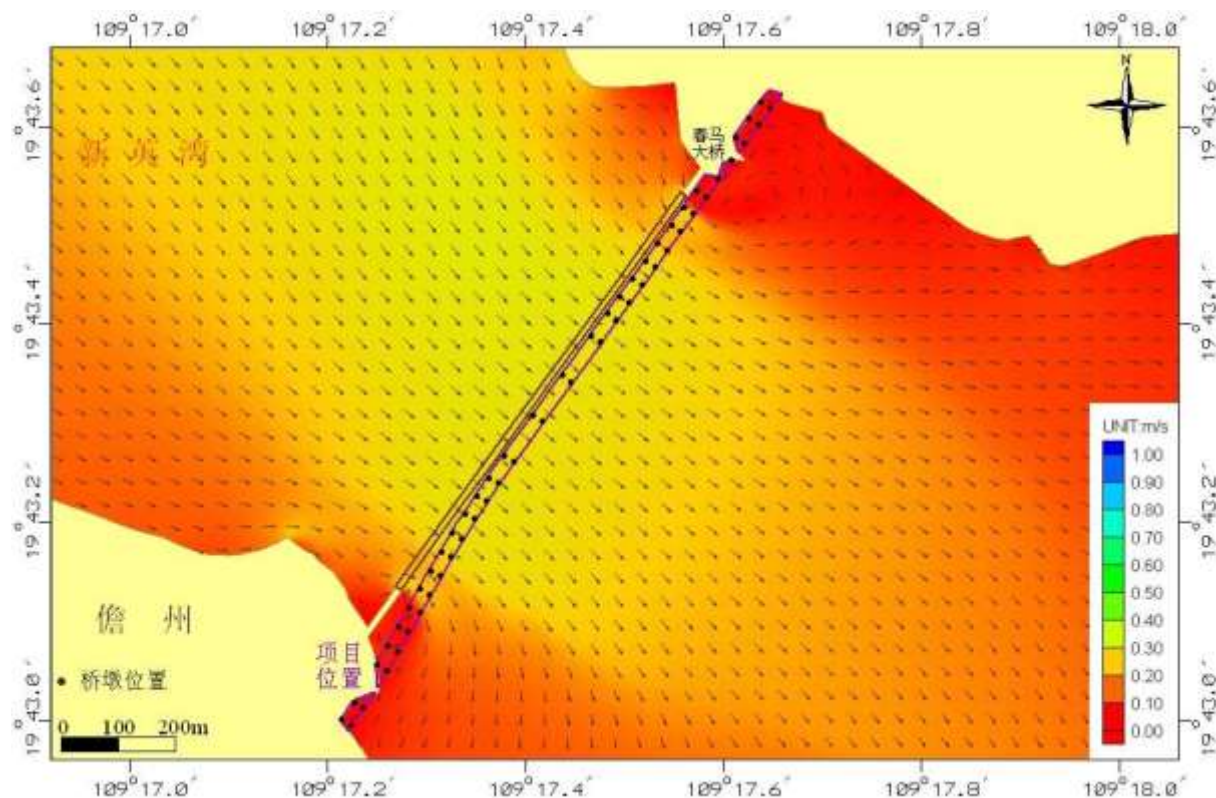
图 4.3-12 工程后项目工程用海区域涨急流场
