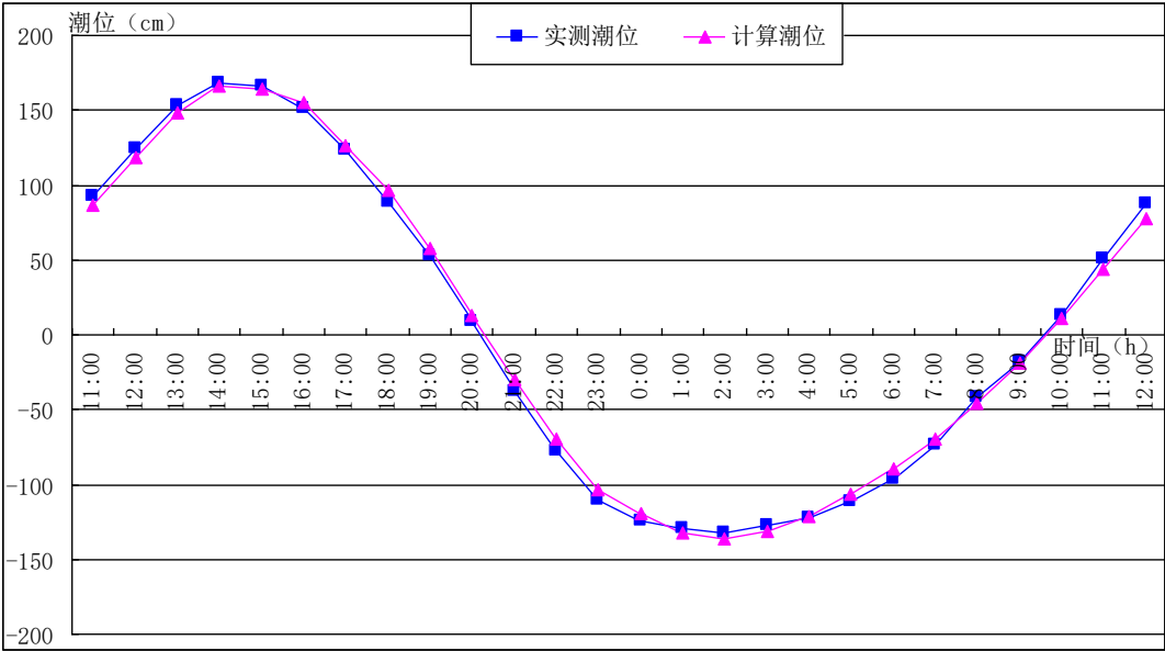
图 4.3-1 潮位验证站 1#站潮位验证(2020 年 9 月 15 日 ~ 16 日)
