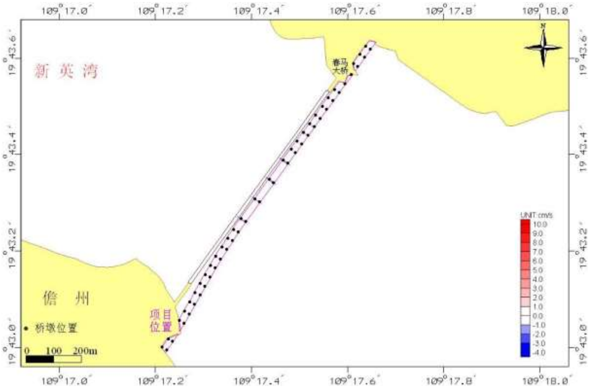
图 4.3-15 工程前后落急时流速大小变化图
