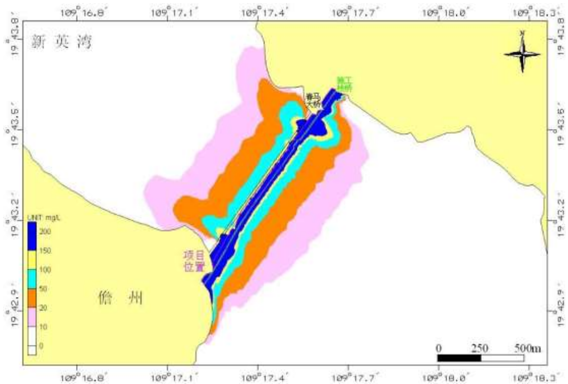
图 4.6-9 整个施工栈桥钢管桩拔除过程中悬浮泥沙增量分布最大包络线图
