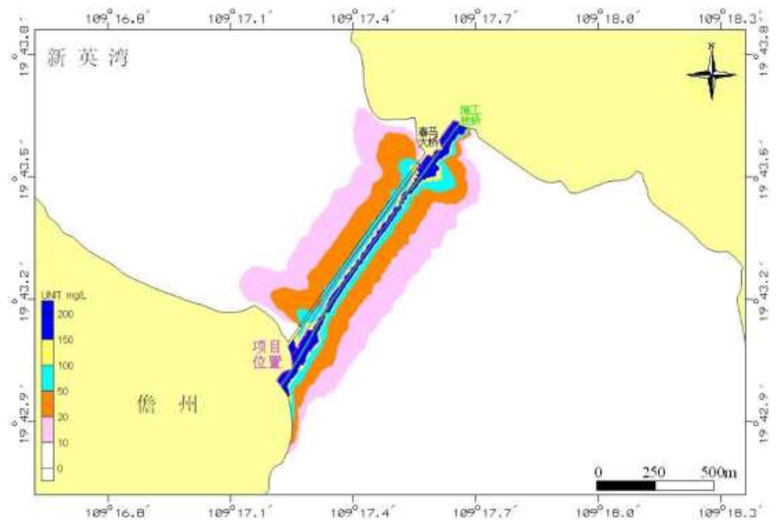
图 4.6-3 整个施工栈桥桩基施工过程中悬浮泥沙增量分布最大包络线图
