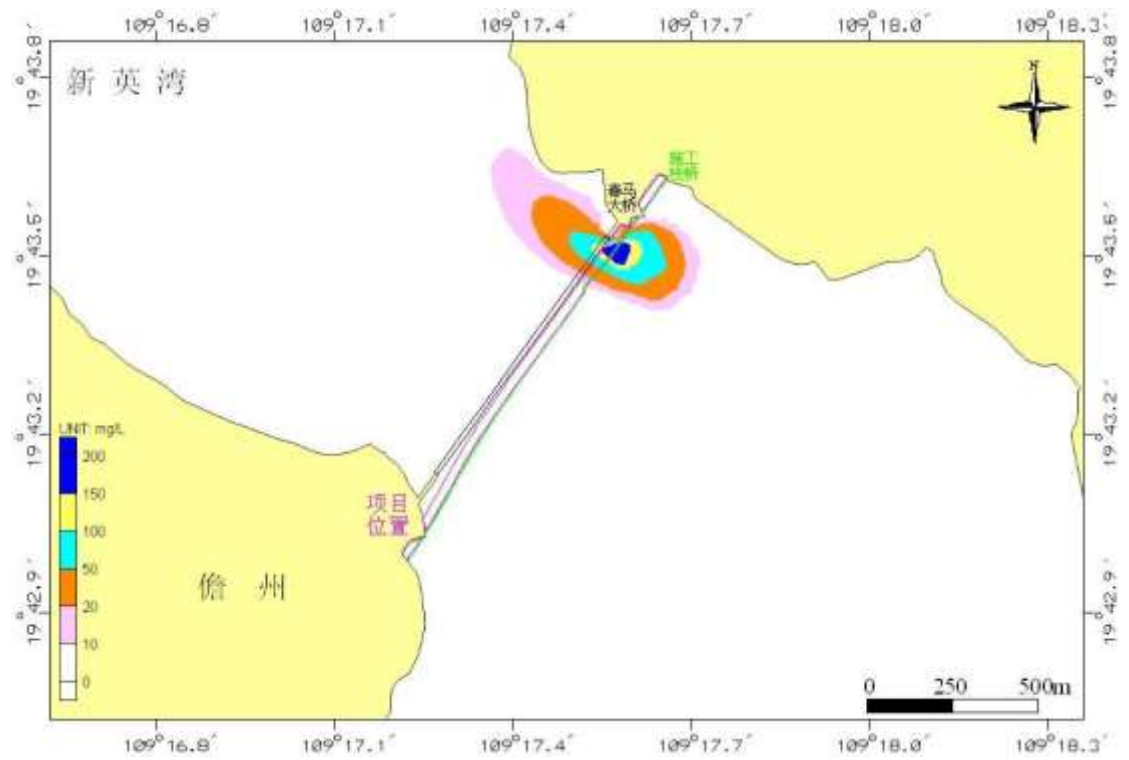
图 4.6-8 源强点 D 钢管桩拔除过程中悬浮泥沙增量分布最大包络线图
