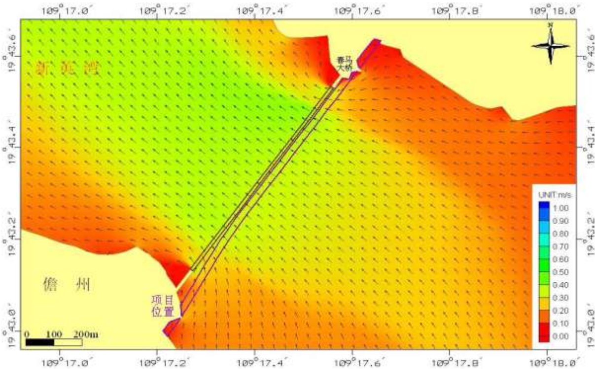
图 4.3-11 工程前项目工程用海区域落急流场
