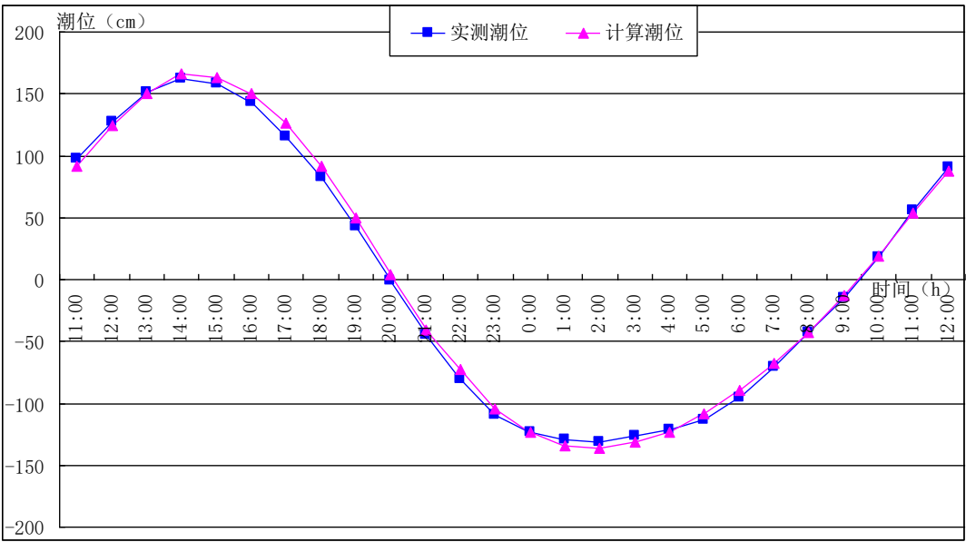
图 4.3-2 潮位验证站 3#站潮位验证(2020 年 9 月 15 日~16 日)
