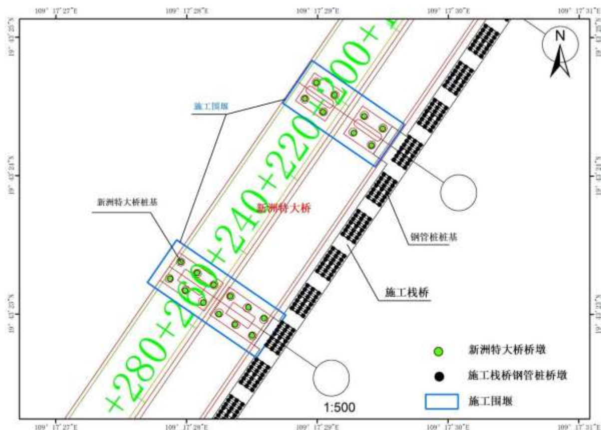
图 4.2-1 新洲特大桥主桥及施工栈桥桥墩、施工围堰位置示意图
