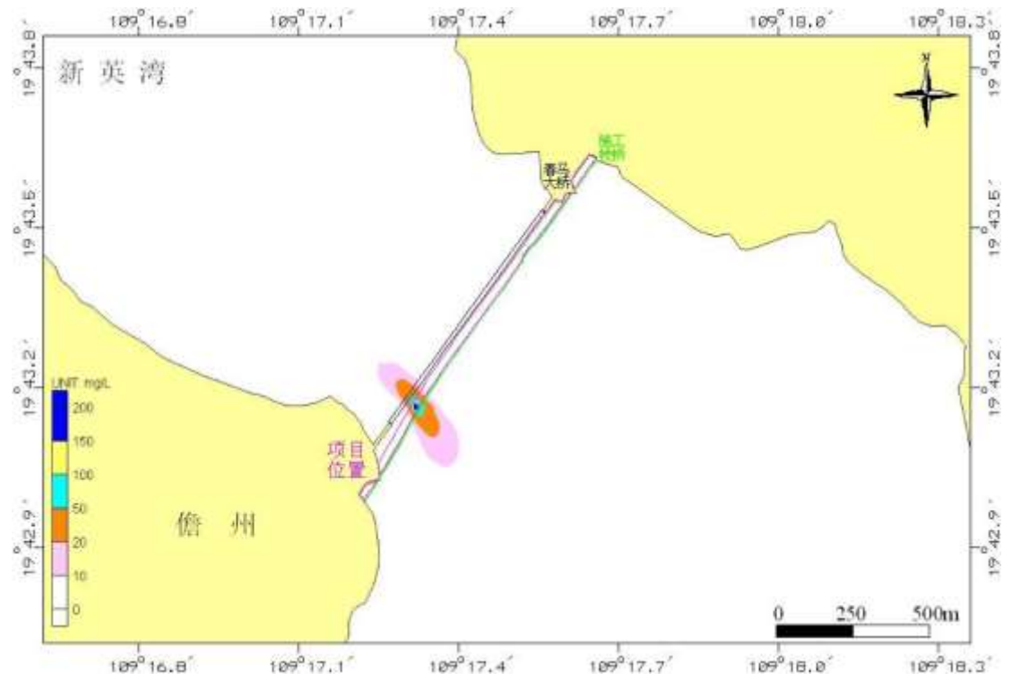
图 4.6-6 源强点 C 围堰拆除过程中悬浮泥沙增量分布最大包络线图
